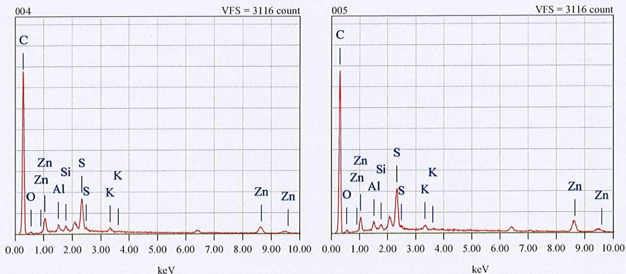
元素分析
