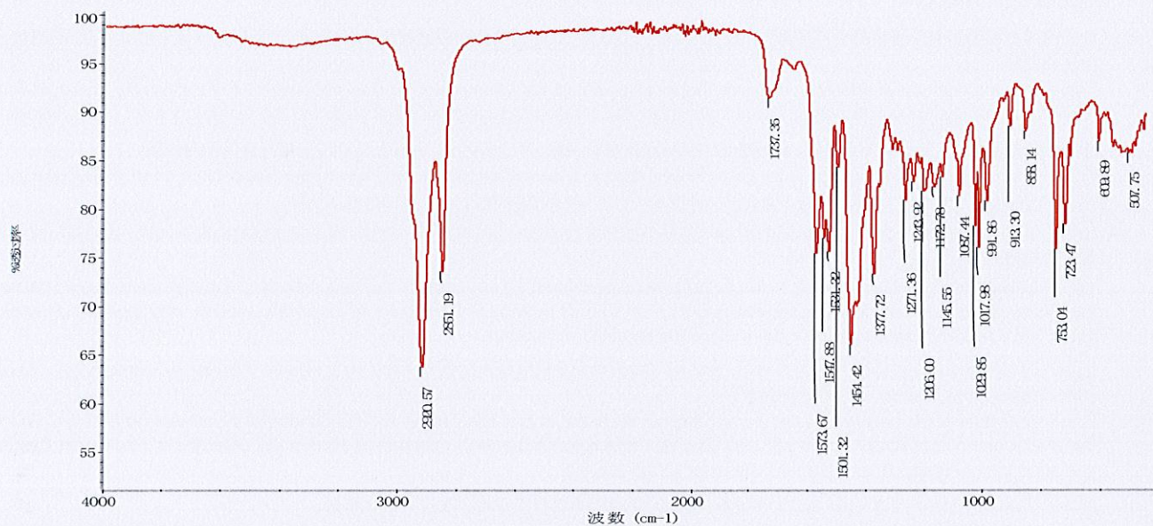
分离产物
